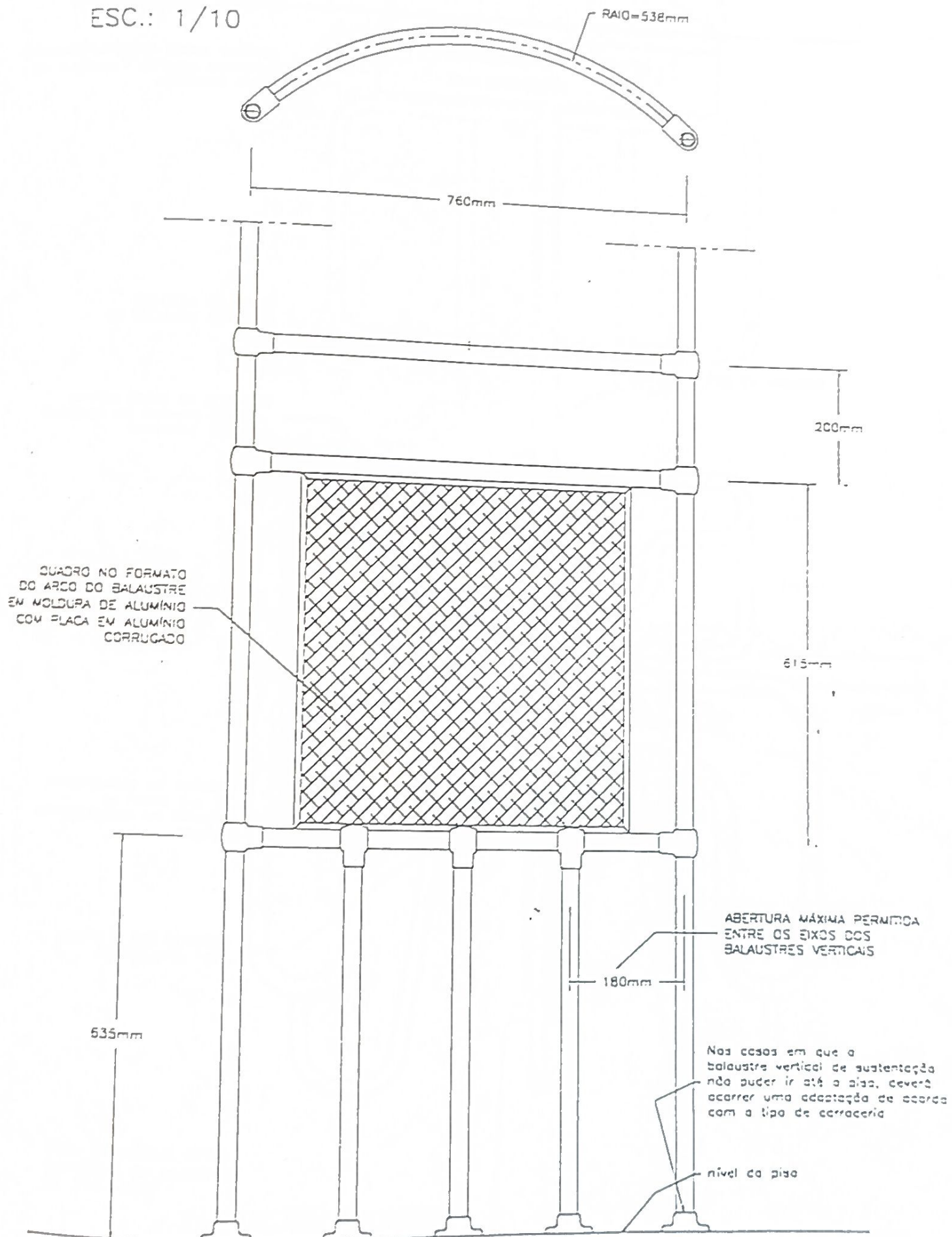
ELEVAÇÃO FRONTAL ESC.: 1/10
